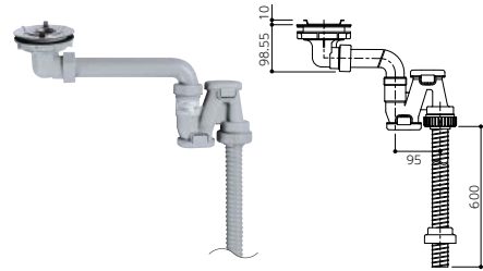
排水トラップセット
