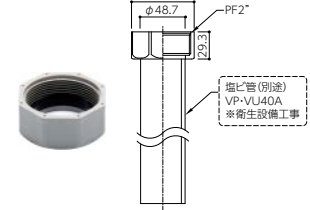
専用排水栓用塩ビ管(VP-VU40A)接続部品 ABH-NAT 袋ナット ABH-PK パッキン 材料設計価格：¥600 材料設計価格：¥200
