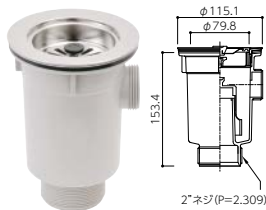
ABH-F50 Flapp/Flapp-R/Flapp-MO専用排水栓 材料設計価格：¥3,700
