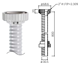
ABH-F800 専用排水ホースセット 材料設計価格：¥2,700
