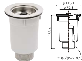
ABH-F50N Flapp-ES専用排水栓 材料設計価格：¥3,200
