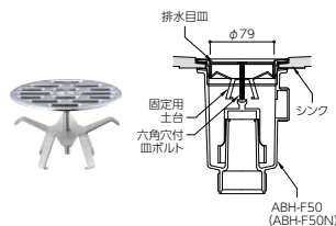
ABH-FK79 固定式目皿 材料設計価格：¥4,300
