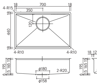
■ JBS-700HL センター排水
