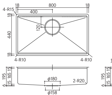
■ JBS-800HL センター排水
