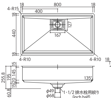
■ JBH-800VB センター排水
