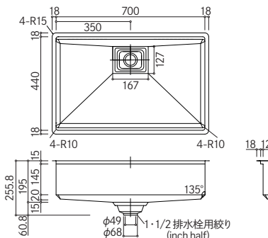
■ JBH-700VB センター排水
